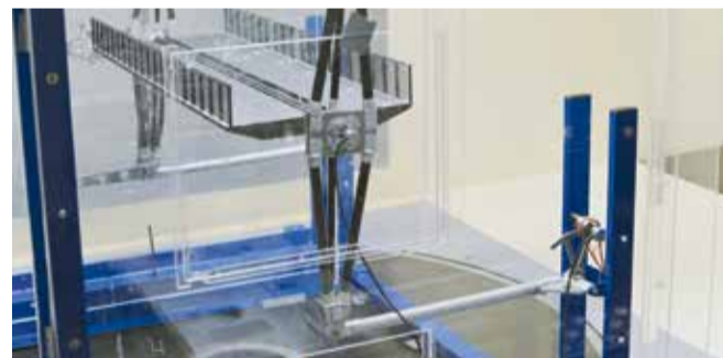
Ispitivanje aerodinamičke stabilnosti modela sekcije mosta u zračnom tunelu Instituta za teorijsku i primjenjenu mehaniku u Pragu
